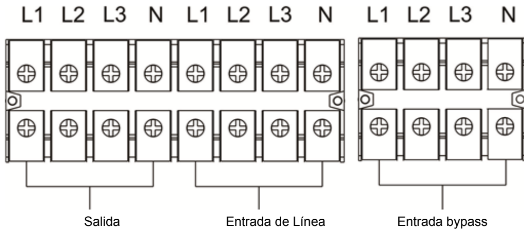
Diagrama de conexiones del bloque de terminales del SAI 10K/20K
