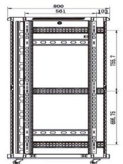
Anclajes trasera
