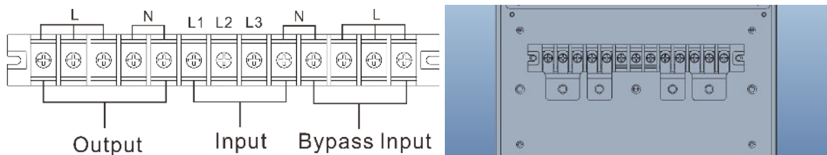
Esquema de ligações 3-1 da folha em cobre de interligação
