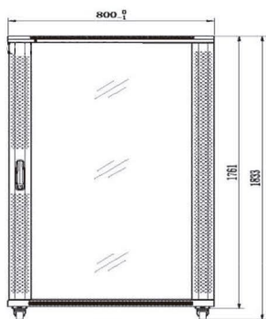
Vista delantera
