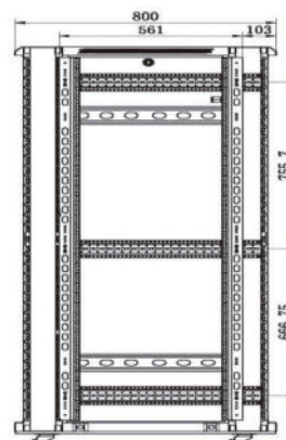
Anclajes trasera
