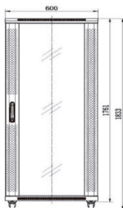
Vista delantera
